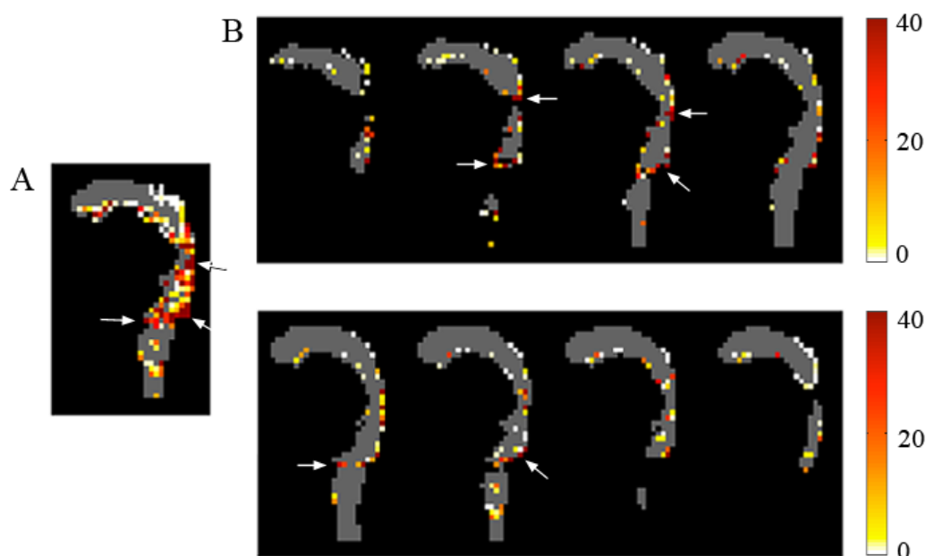
FIGURE 5.2.13 : Cartes de dépôt de fer sur les parois du fantôme bouche-trachée calculées par CFD (en \mu\text{g}_{\text{Fe}}\cdot\text{voxel}^{-1} ). (A) Projection 2D sur l'ensemble du volume. (B) Représentation des huit coupes centrales.
