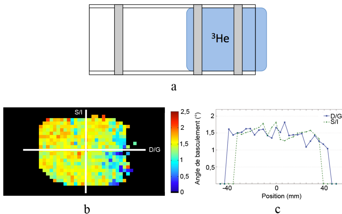
FIGURE 4.2.4 : Carte de distribution des angles de basculement (carte de B_1 ) pour un fantôme placé dans l'antenne petit animal obtenue sur 64 dynamiques : FOV = (288 \times 96 \times 96) \text{ mm}^3 , \text{voxel} = (4 \times 4 \times 4) \text{ mm}^3 , \text{TE/TR} = 1,73/4 \text{ ms} , \alpha = 2^\circ . (a) Position du fantôme dans l'antenne. (b) Coupe coronale centrale, \alpha_{\text{moyen}} = 1,5^\circ \pm 0,17^\circ . (c) Deux profils d'angles de basculement sélectionnés sur la carte (b) (S/I supérieur, inférieur et D/G droite, gauche).
