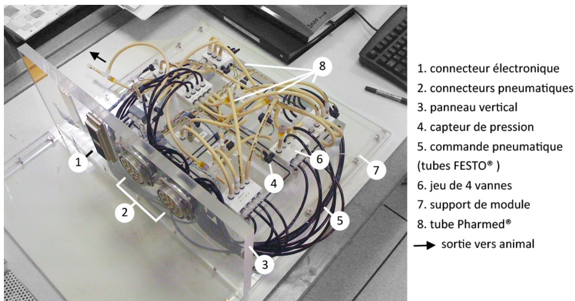
FIGURE 6.1.14 : Module d'administration de SAGAS après assemblage.
